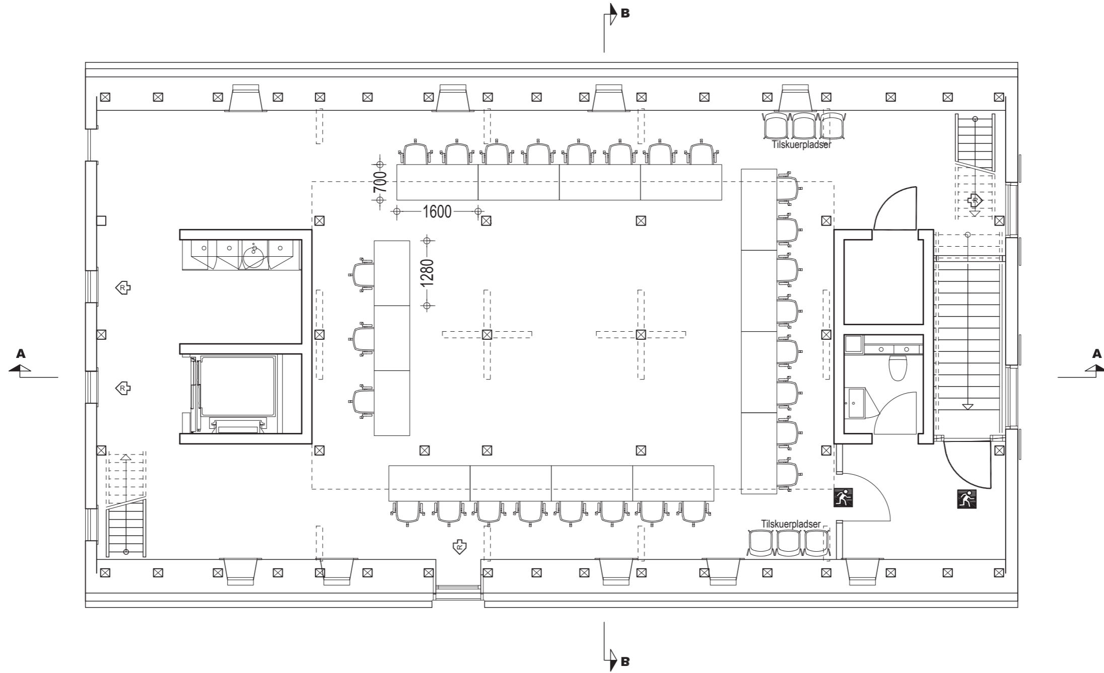
1. Salsplan - Byrådssal med 27 siddepladser Mål 1:75
