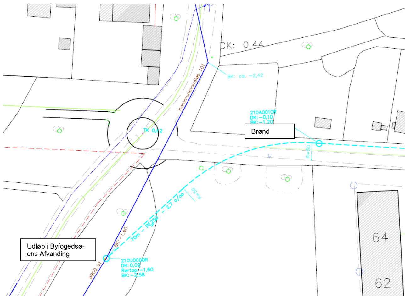
Bilag 3: Situationsplan, tilslutning til Byfogedsøens Afvanding
