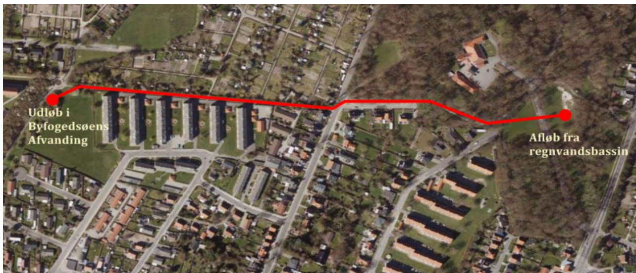
Bilag 2: Placering af afløbsledning fra forsinkelsesbassin til udløb i Byfogedsøens Afvanding
