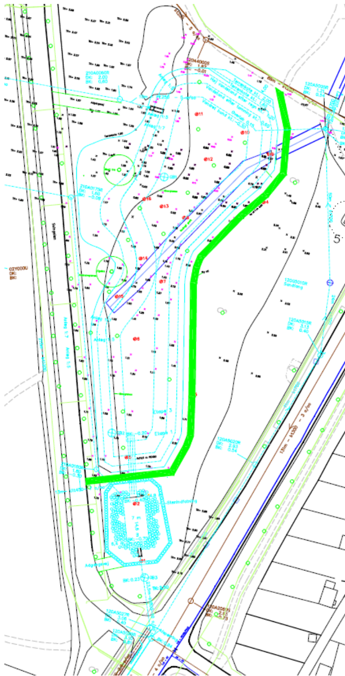
Bilag 4: Situationsplan, regnvandsbassin
