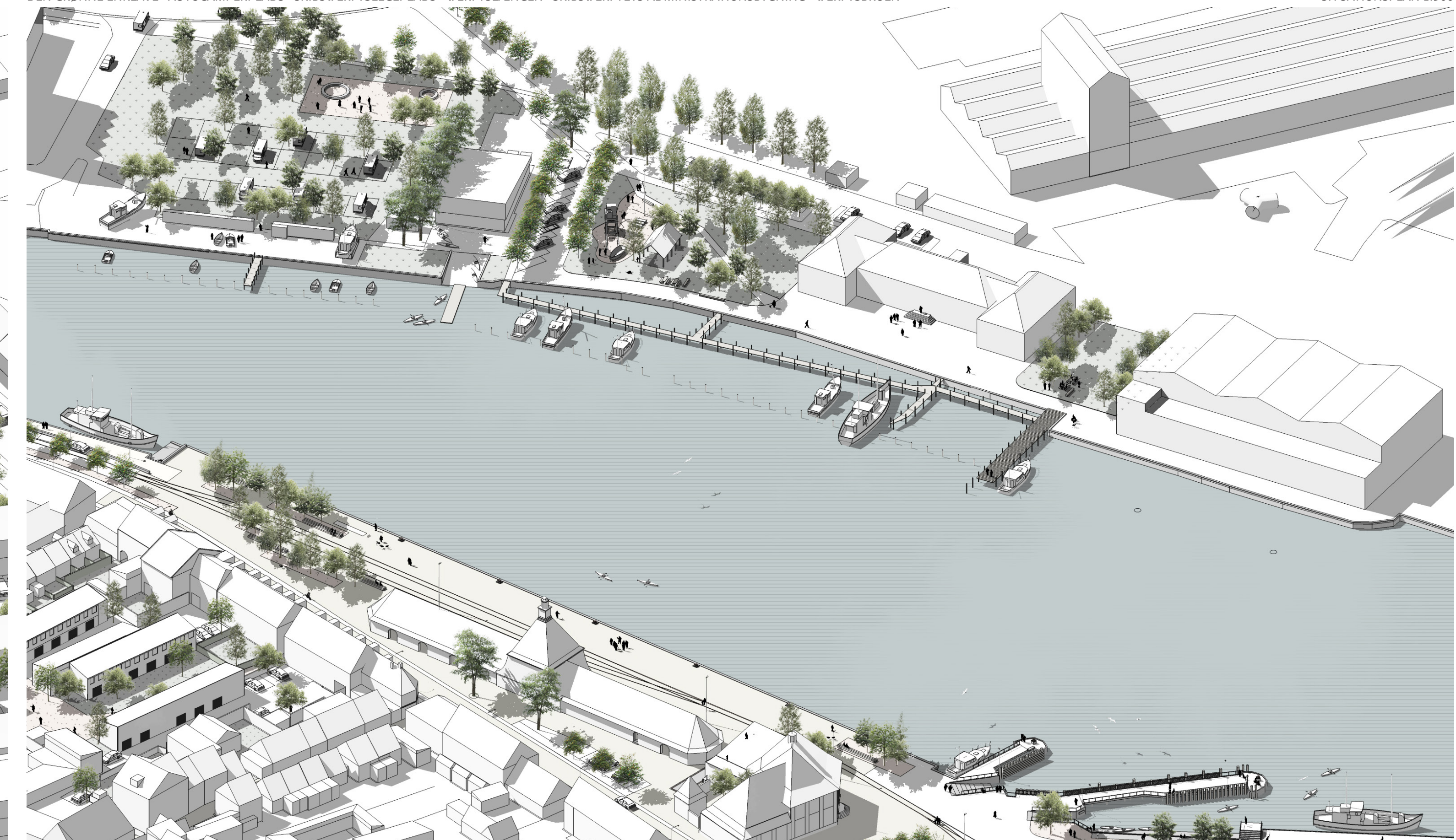
LILLE NYBRO - NYBROTTRAPPEN - MØRTELKAJ - MØRTELPLADSEN - SYKAKAJEN DEN GRØNNE ENKLE - AUTOCAMPERPLADS - SKIBSVÆRFTSLEGEPLADS - VÆRFTSLÆNGEN - SKIBSVÆRFTETS ADMINISTRATIONSBYGNING - VÆRFTSBROEN SITUATIONSPLAN 1:500
